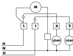
W200 (DPST)
