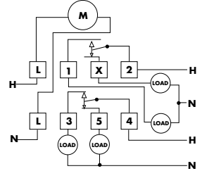
W220 (DPDT)
