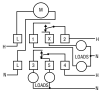
DPDT - 7220
