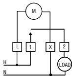
SPST - 7100
