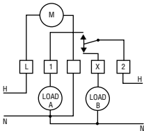
SPDT - 7120
