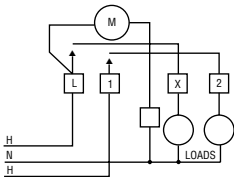
DPST - 7200
