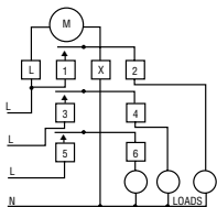
3PST - 7300
