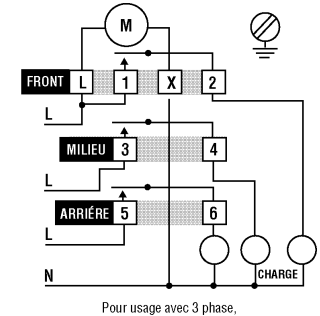
Pour usage avec 3 phase, alimentation de 4-wire, 120/208V c.a.
