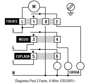
Diagrama Para 3 Fases, 4 Hilos 120/240V~.
