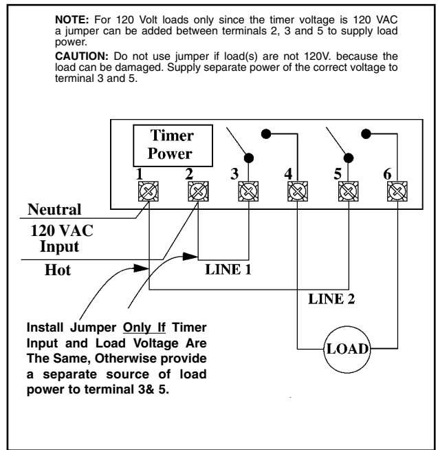
FIG. #4 ET103C DPST
