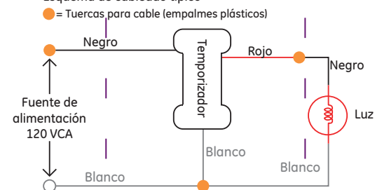
Esquema de cableado típico
