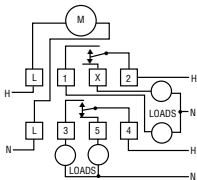
DPDT - 7220
