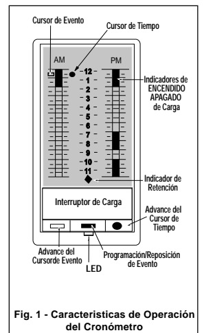
Fig. 1 - Características de Operación del Cronómetro
