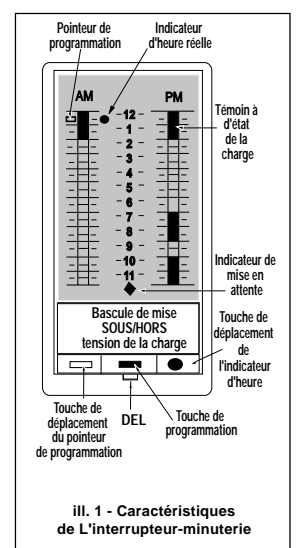
Ill. 1 - Caractéristiques de L'Interrupteur-minuterie
